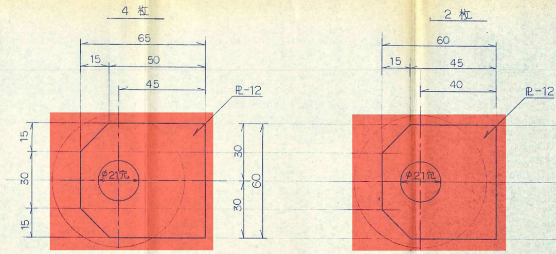
ローラー取付板 s=1/1
